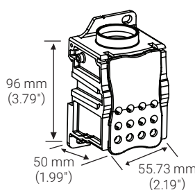
UD-400112AL & UD-400112CU 400 A – IEC 335 A – cULus 1 câble – 12 câbles
